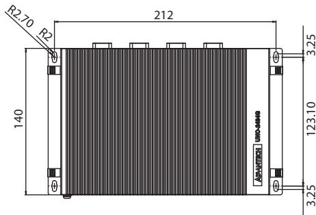
UNO-2484G V2 Single stack
